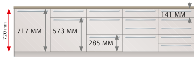
HAUTEUR STANDARD : 720 MM DE HAUTEUR, AVEC POIGNÉE TRAME DE 5
