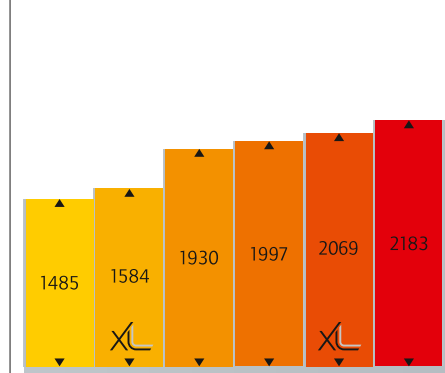
82 6 HAUTEURS D'ARMOIRE
