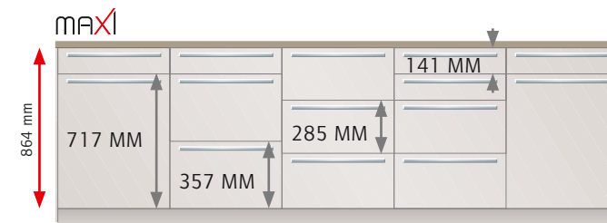
HAUTEUR MAXI : 864 MM DE HAUTEUR, AVEC POIGNÉE
