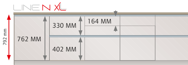
HAUTEUR XL : 792 MM DE HAUTEUR, SANS POIGNÉE
