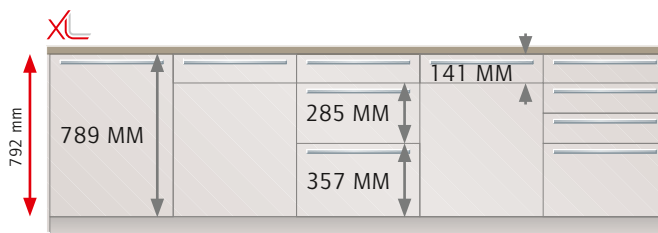
HAUTEUR XL : 792 MM DE HAUTEUR, AVEC POIGNÉE
