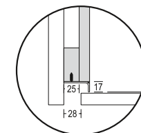
Poignée encastrable fin de ligne
